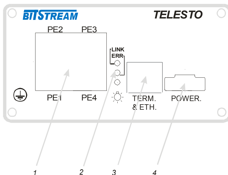
Rys. 2. Panel przedni urządzenia
