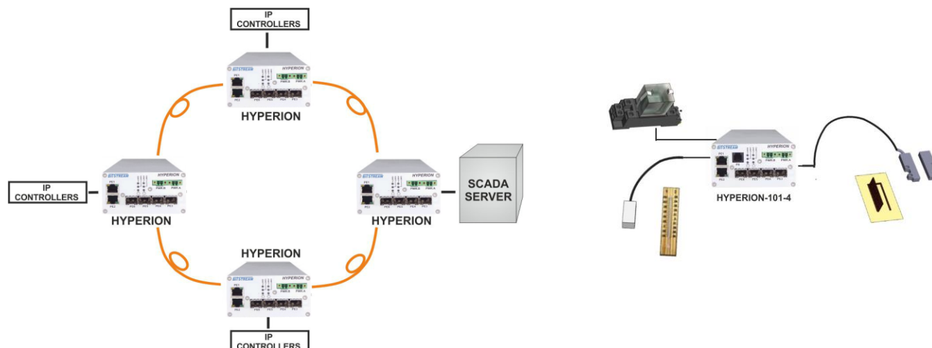
Rys. 1. Przykładowa aplikacja. Zapewnienie łączności pomiędzy kamerami a systemem monitorującym. Praca w warunkach przemysłowych pozwala instalować urządzenia w obiektach narażonych na trudne warunki pracy. Dodatkowo można podłączyć szereg czujników.
